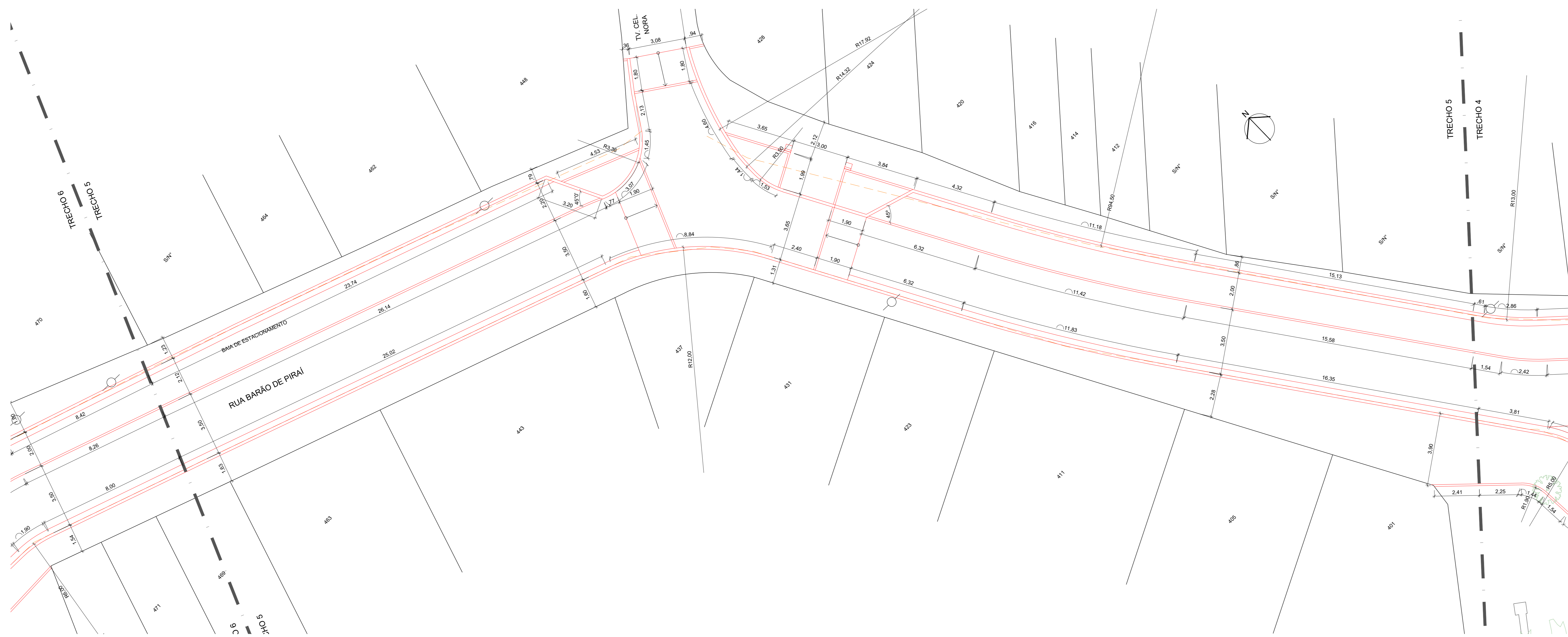
01 PLANTA TRECHO 5 ESCALA 1:1100
