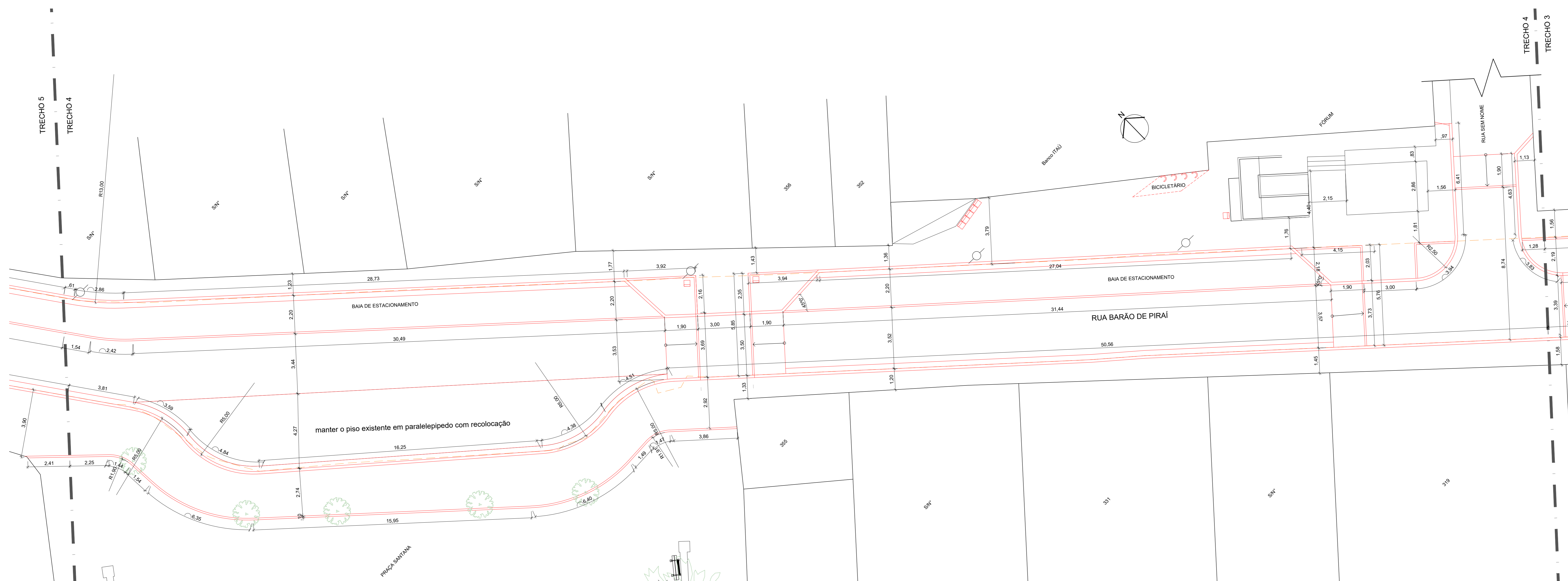
02 PLANTA TRECHO 4 ESCALA 1/100
