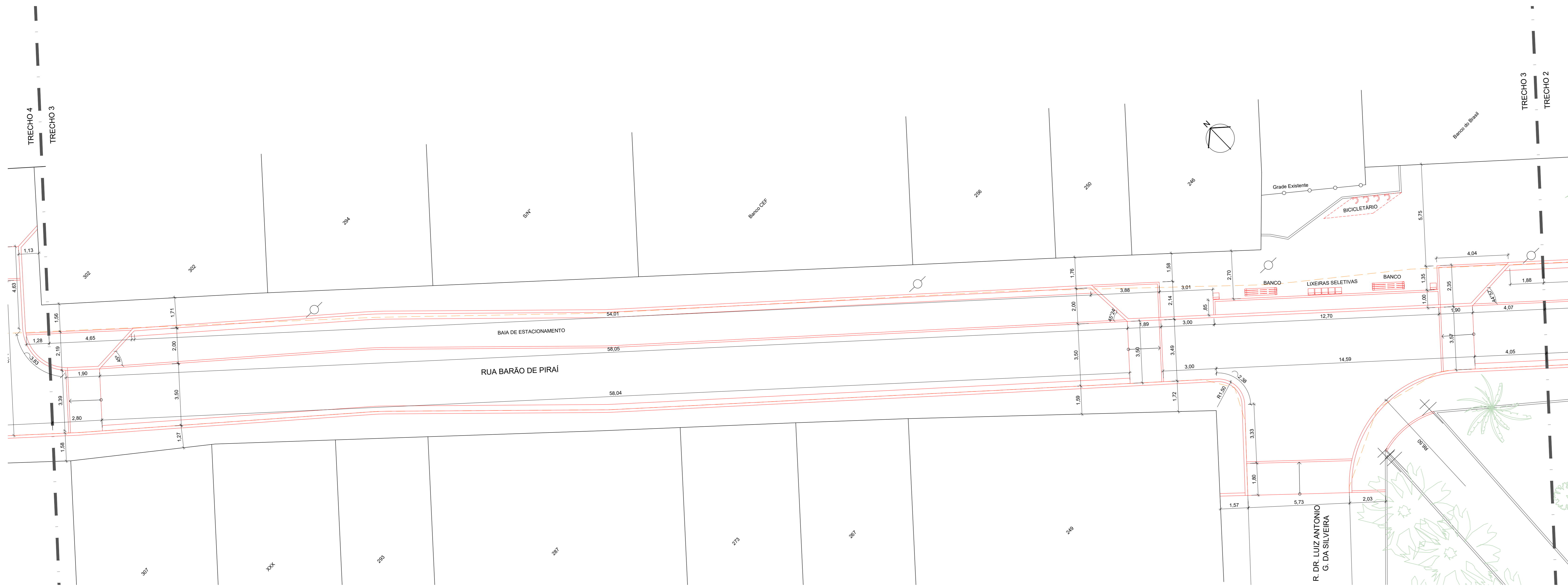
01 PLANTA TRECHO 3 ESCALA 1/100
