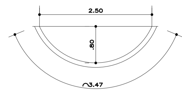
DETALHE - CANTEIRO ESC.: 1/50
